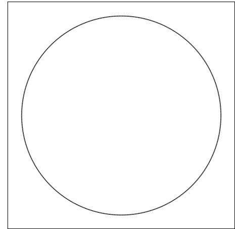
Figura 3.1: Circunferência.
